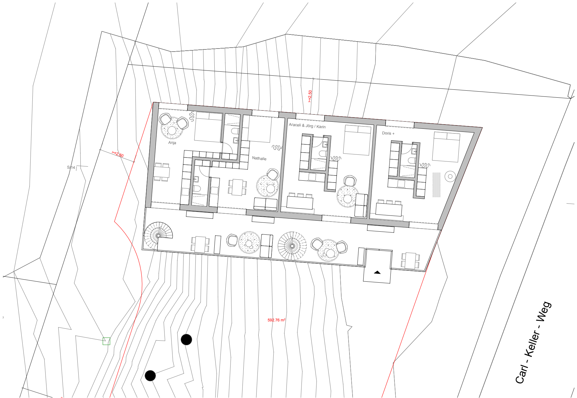
Erdgeschoss -1,00
