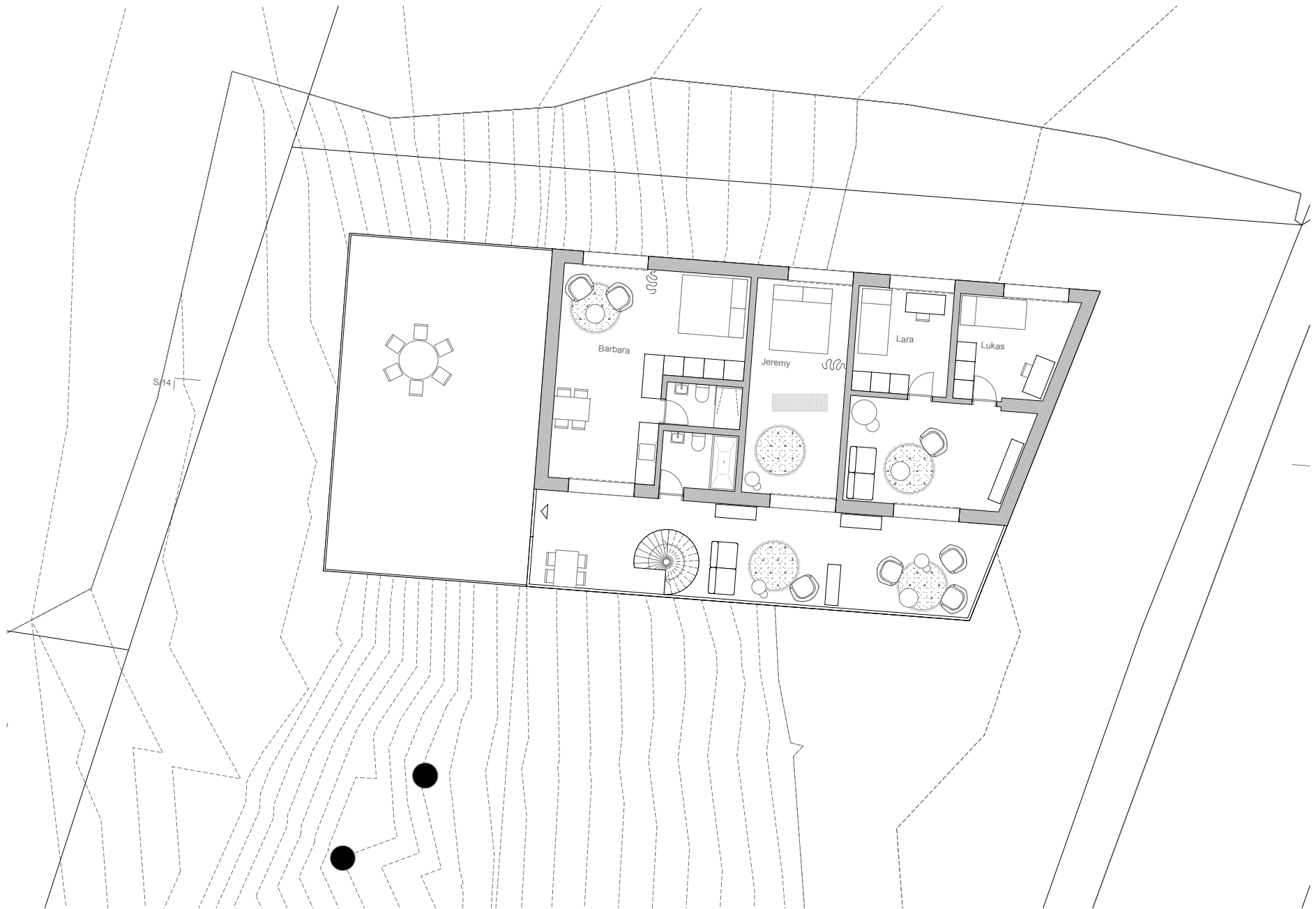
Obergeschoss +3,00
