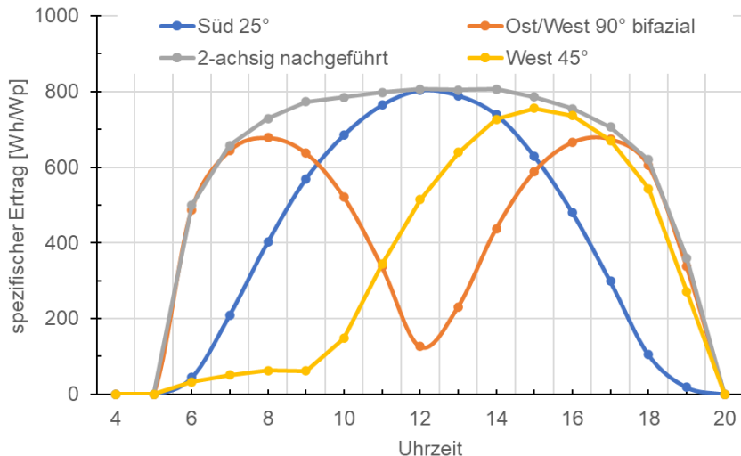
Abbildung 51: Stomertragsprofile von PV-Kraftwerken in verschiedenen Montagevarianten, berechnet online mit https://re.jrc.ec.europa.eu/pvg_tools für einen überwiegend klaren Maitag am Standort Freiburg, ohne Verschattungseffekte, Bifazialitätsfaktor 100%.
