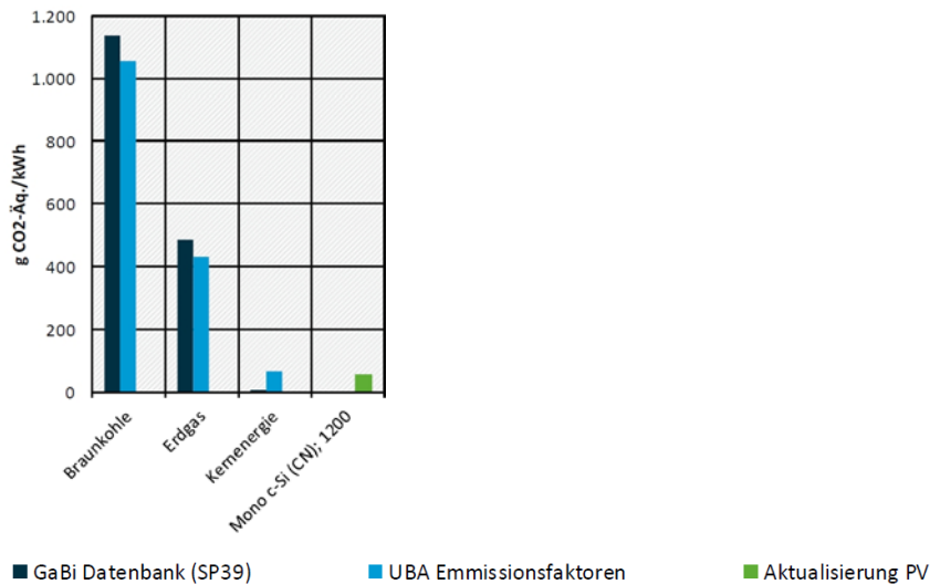
Abbildung 42: Treibhauspotenzial verschiedener Stromerzeugungstechnologien [UBA7].
