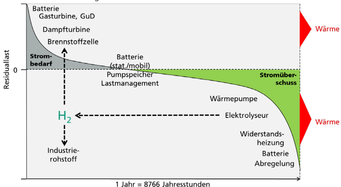
Abbildung 49: Schematische Darstellung einer Residuallastkurve für Deutschland bei Stromversorgung mit 100 % EE.
