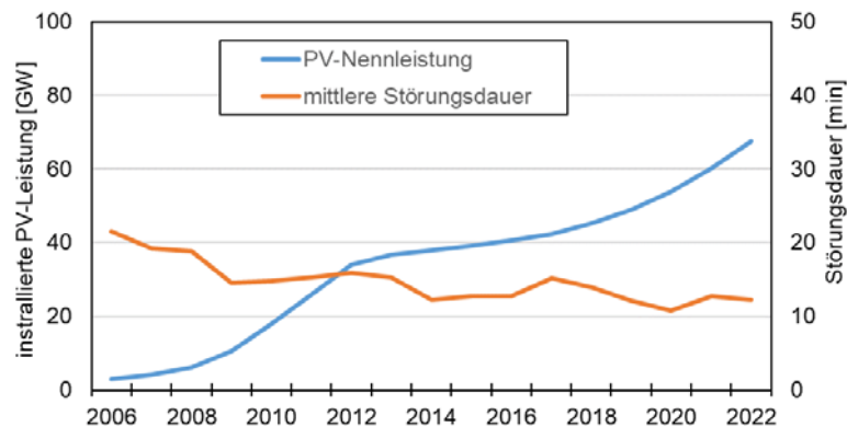
Abbildung 25: System Average Interruption Duration Index (SAIDI) für die Nieder- und Mittelspannung, Daten aus [BNA2].
