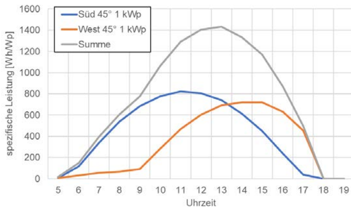
Abbildung 35: Stundenprofil der Stromproduktion an einem klaren Apriltag für verschiedene Dachausrichtungen bei 45° Dachneigung, unverschattet, Standort Freiburg, berechnet online mit https://re.jrc.ec.europa.eu/pvg_tools/en/ .
