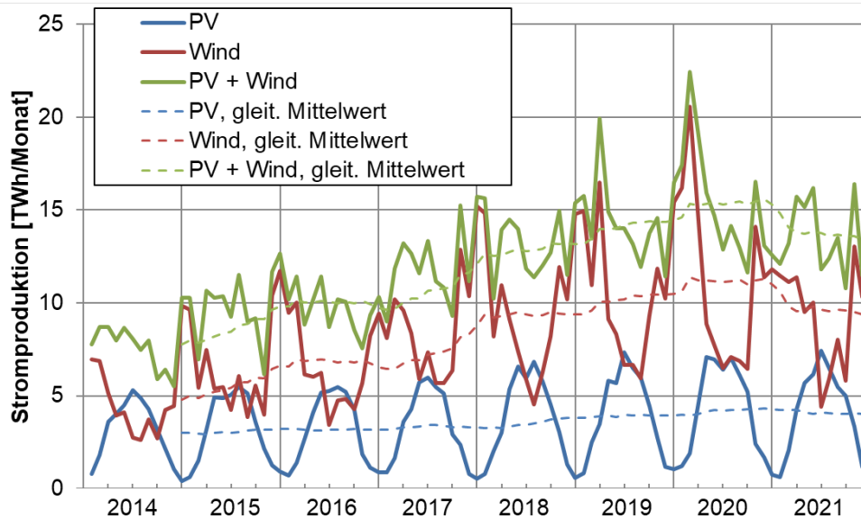
Abbildung 23: Monatssummen PV- und Windstromproduktion, Daten aus [ISE4].
