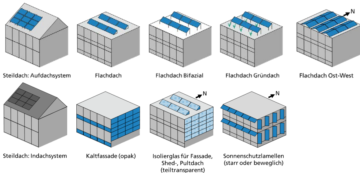
Abbildung 29: PV-Lösungen für Dach und Fassade (oben: Aufdachsysteme, unten: Integrierte PV).
