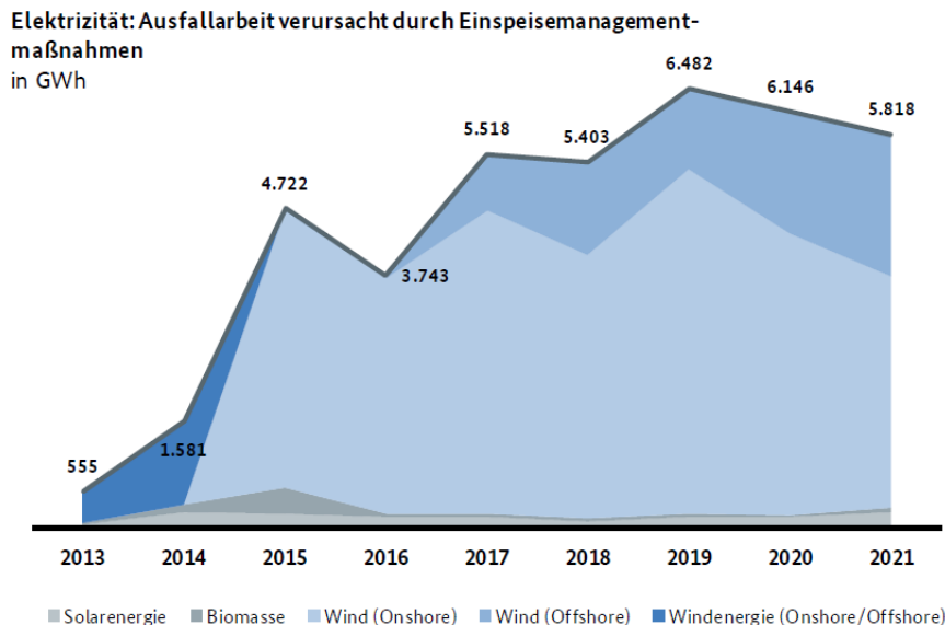
Abbildung 20: Abgeregelte elektrische Energie [BNA2].
