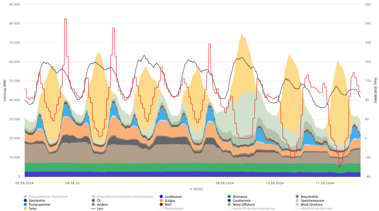
Abbildung 24: Beispiel für den Verlauf von Börsenstrompreisen, konventioneller und regenerativer Stromerzeugung der 32. Kalenderwoche 2024 [ISE4].
