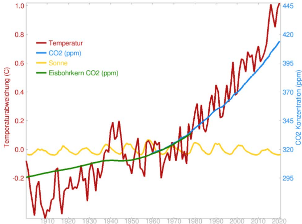
Abbildung 39: Entwicklung der atmosphärischen CO 2 -Konzentration, der mittleren globalen Temperaturveränderung und der Sonnenaktivität ( http://herdsoft.com/climate/widget/ ).
