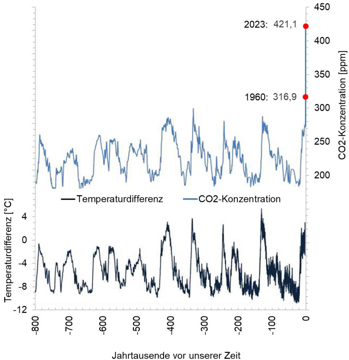
Abbildung 40: Schätzungen der atmosphärischen CO 2 -Konzentration und der Temperaturdifferenz in der Antarktis auf Basis von Eisbohrkernen [EPA]; Rot: zwei neuere CO 2 -Messwerte des Mauna Loa Observatory [ https://www.esrl.noaa.gov/gmd/ccgg/trends/data.html ].
