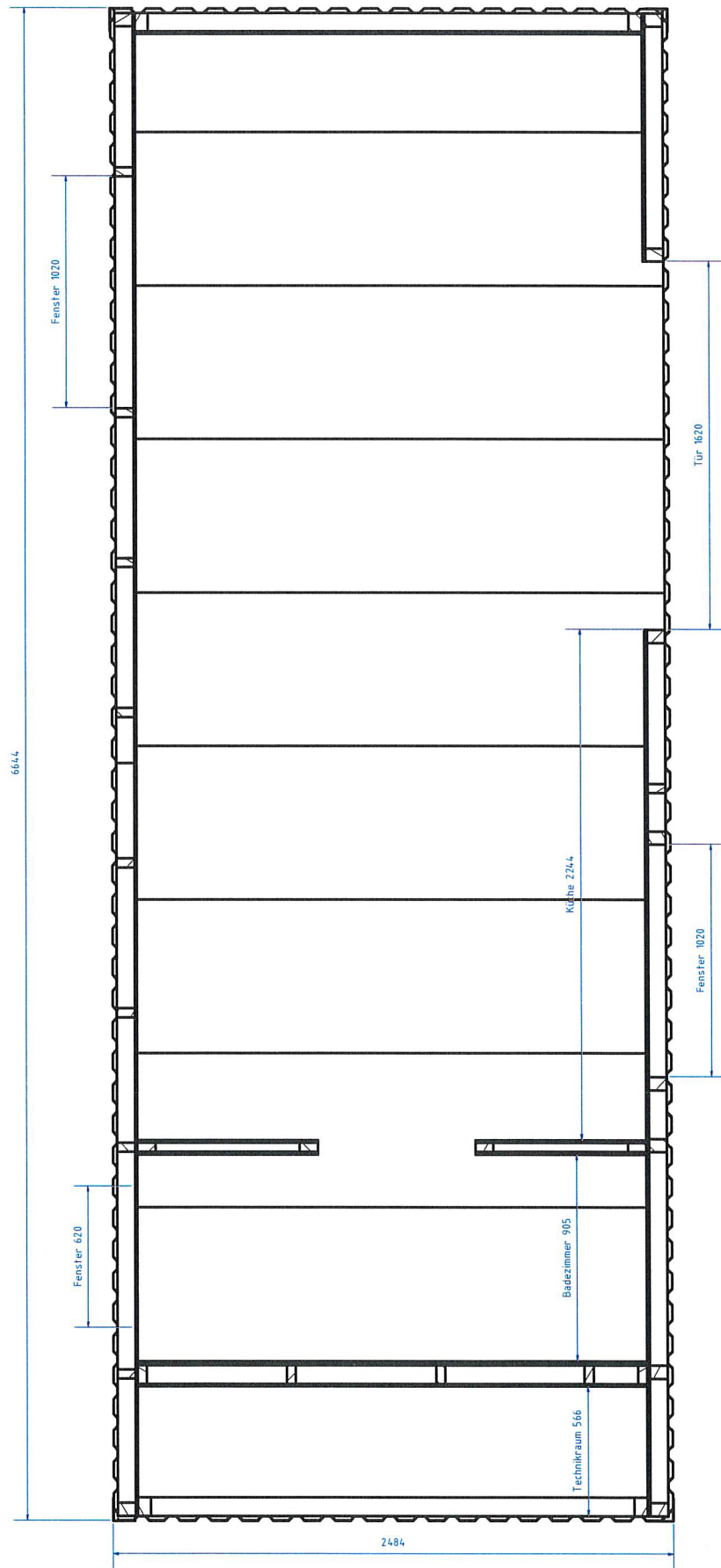
A-A ( 1 : 20 )
